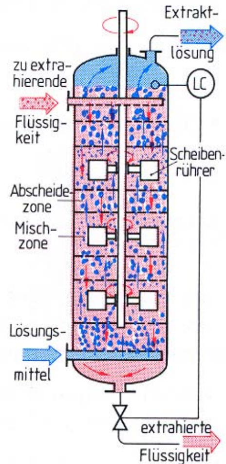
Bild 345/2: Kolonnen mit bewegten Einbauten
