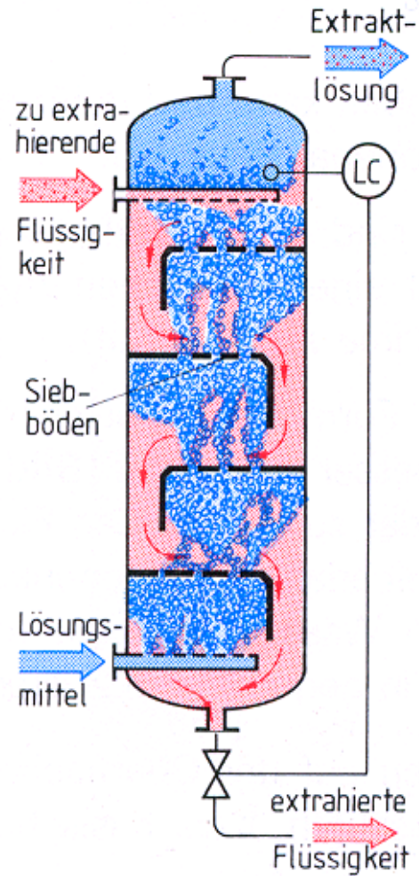
Bild 345/1: Kolonnen mit feststehenden Einbauten
