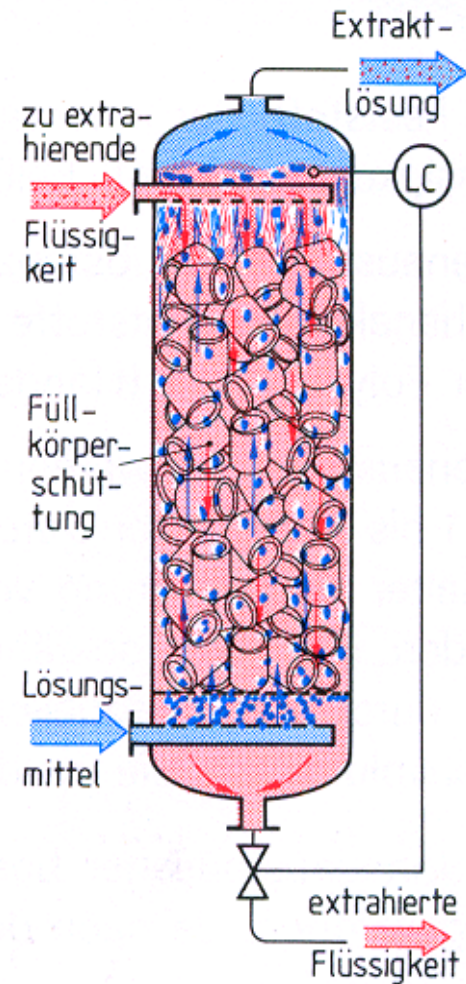
Bild 345/1: Kolonnen mit feststehenden Einbauten
