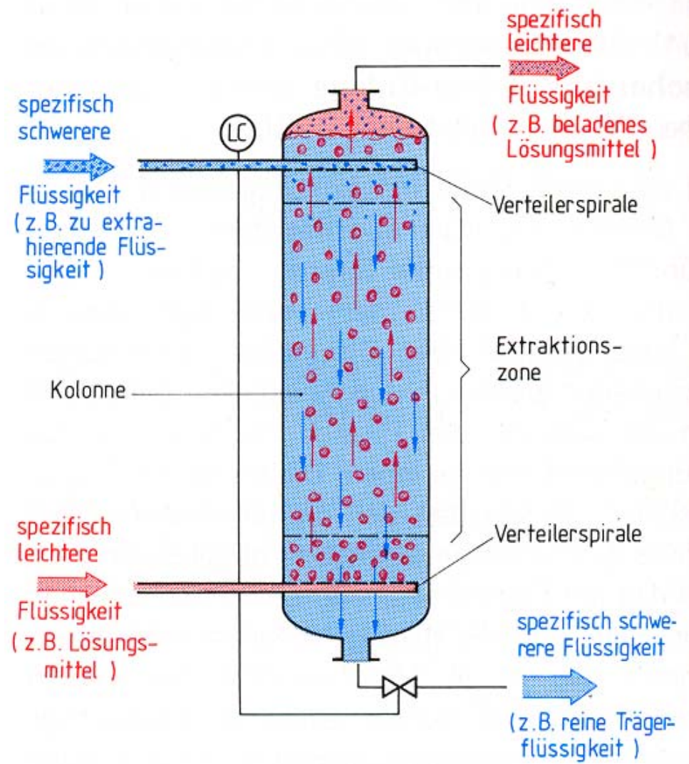
Bild 344/2: Extraktionskolonne (schematisch)
