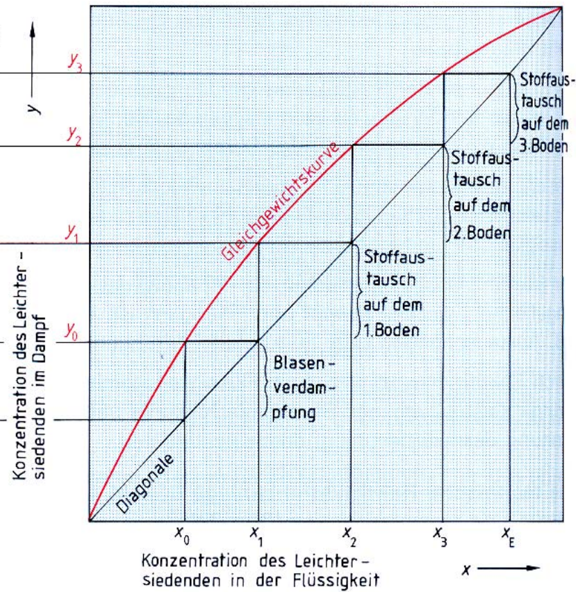
Bild 322/2: Konzentrationsverlauf beim Rektifizieren im Gleichgewichtsdigramm (bei totalem Rücklauf)
