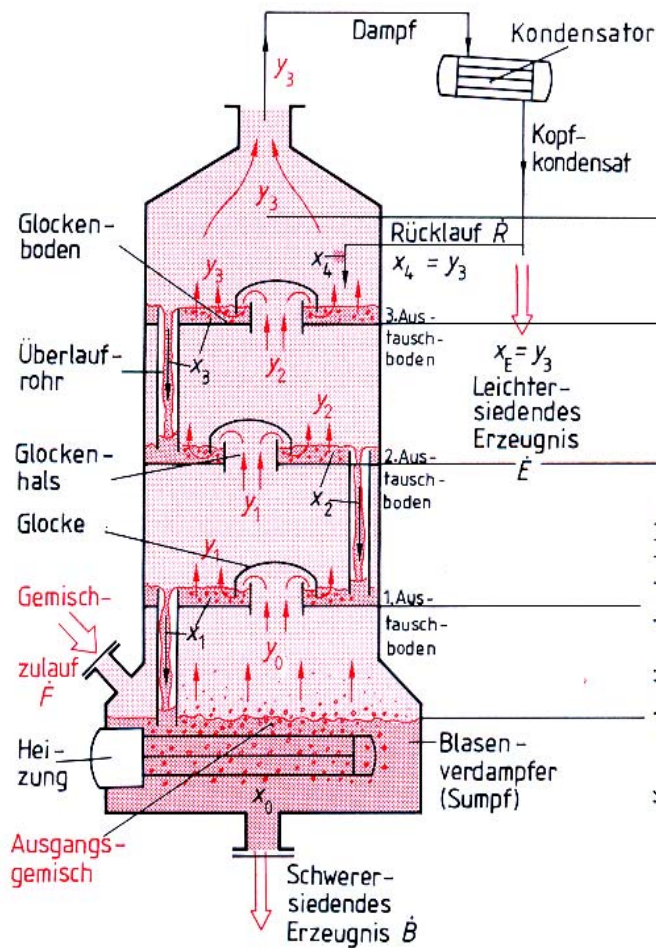
Bild 322/1: Vorgänge in einer Glockenbodenkolonne
