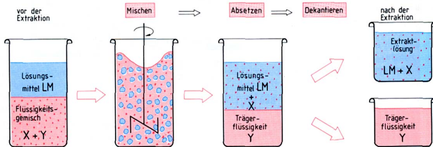
Bild 342/1: Einzelvorgänge bei der Flüssig-Flüssig-Extraktion
