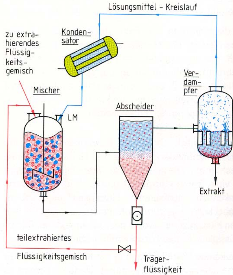
Bild 343/1: Einstufige Mischer-Abscheider-Extraktionsanlage
